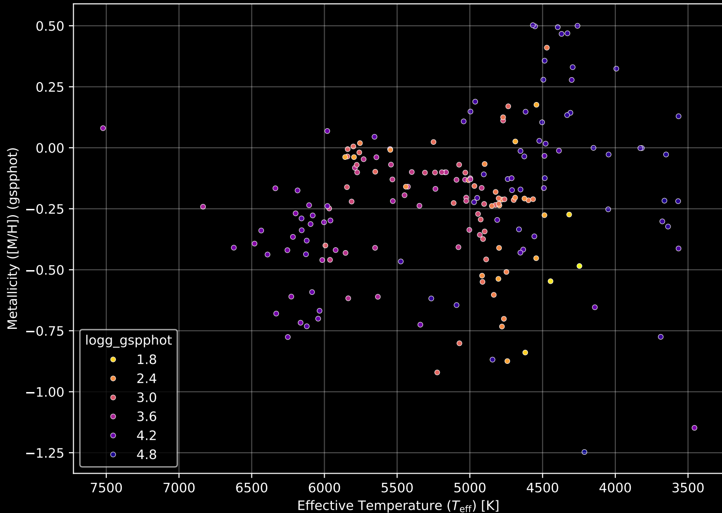
APOGEE DR17 Field: [340+60] Stellar Population Parameters (n= 189)
